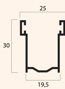
Guida in alluminio estruso A30 19,5 x 30 mm
