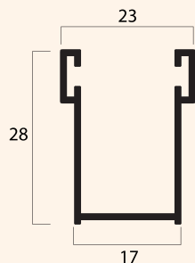
Guida in alluminio estruso A28 17 x 28 mm
