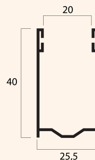
Guida in alluminio estruso A40 25,5 x 40 mm
